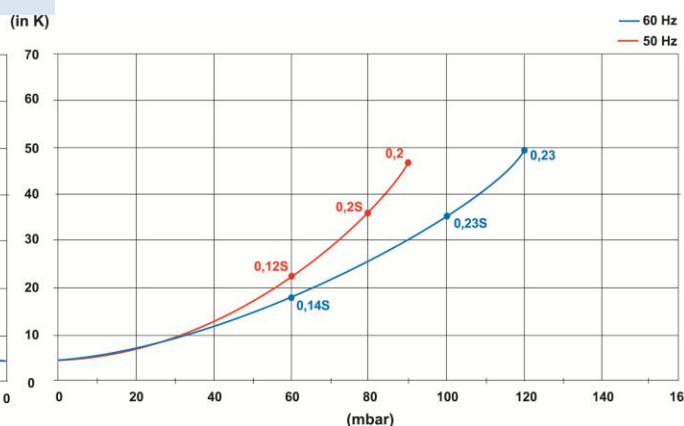
Hausse de température de l'air véhiculé / Temperature rise on the exhaust air
